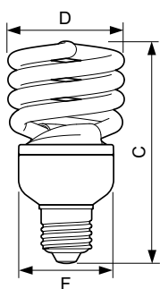
EconomyTwister 23W CDL E27 1PF/6
